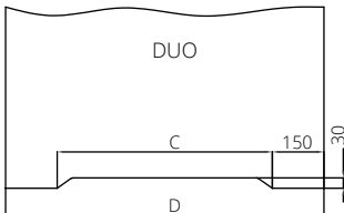
podcięcie wentylacyjne w skrzydłach bezprzylgowych z kolekcji DUO - dopłata powierzchnie fornirowane 50/61,50 - dopłata powierzchnie syntetyczne/malowane 35/43,05
