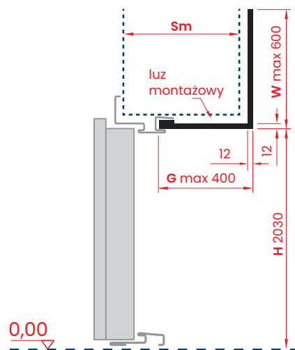
PRZEKRÓJ PIONOWY
