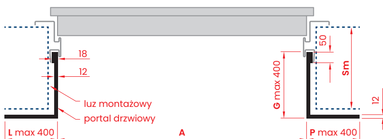
PRZEKRÓJ POZIOMY
