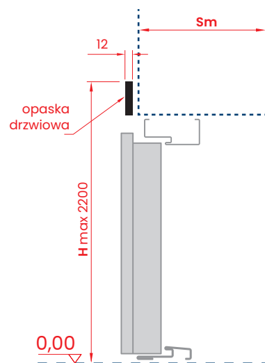
PRZEKRÓJ PIONOWY
