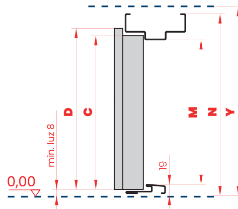
PRZĘKRÓJ PIONOWY
