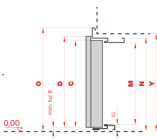
PRZEKRÓJ PIONOWY
