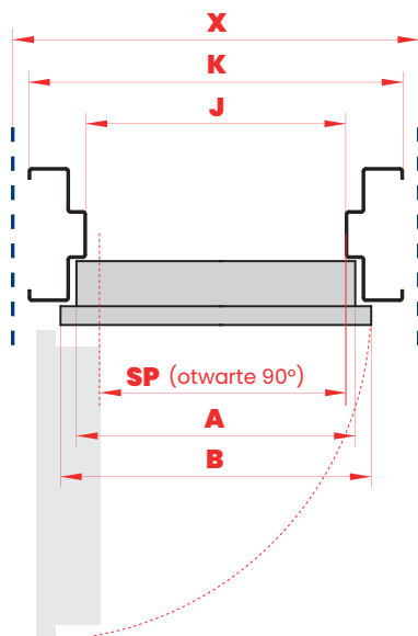
PRZĘKRÓJ POZIOMY
