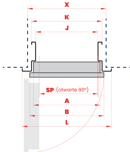
PRZEKRÓJ POZIOMY
