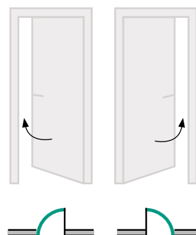
DRZWI Z ODWROTNĄ PRZYLGĄ SKRZYDŁO LEWE SKRZYDŁO PRAWE
